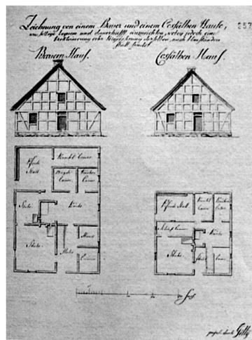
Ryc. 10. David Gilly, projekty chałup chłopskich, 1784, rysunek piórem (Helmigk 1938: 55)
