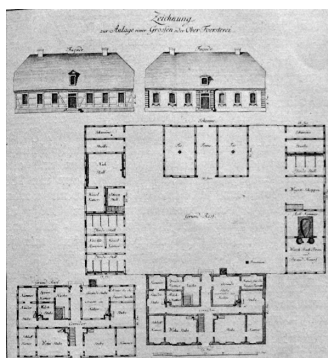
Ryc. 12. Projekt leśniczówki z 1781 roku, rysunek piórem (Helmigk 1938: 53)
